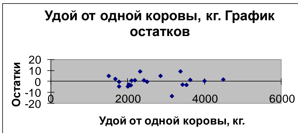
Графики остатков
