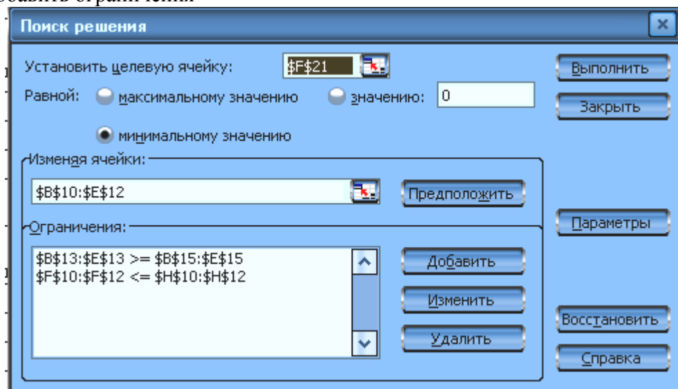
Рисунок 2 - Диалоговое окно надстройки Поиск решения
